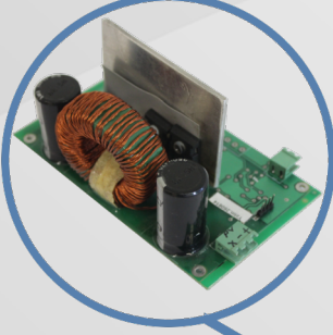
MPPT Solar Kontrol Kartı
