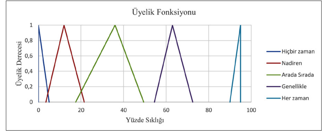
Şekil 6. Üyelik Fonksiyonu
